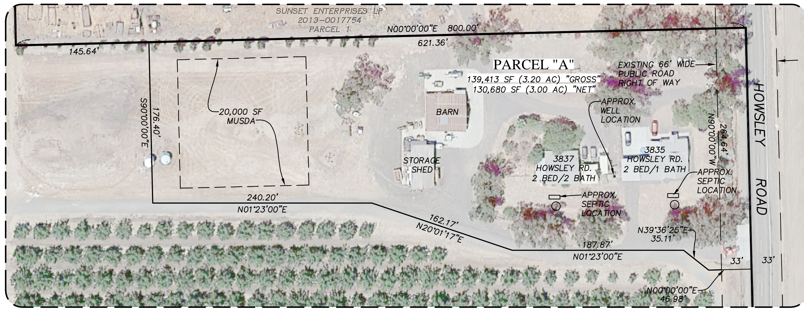
DETAIL "A" SCALE: 1" = 60'
